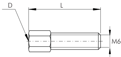
Stellschraube M6
